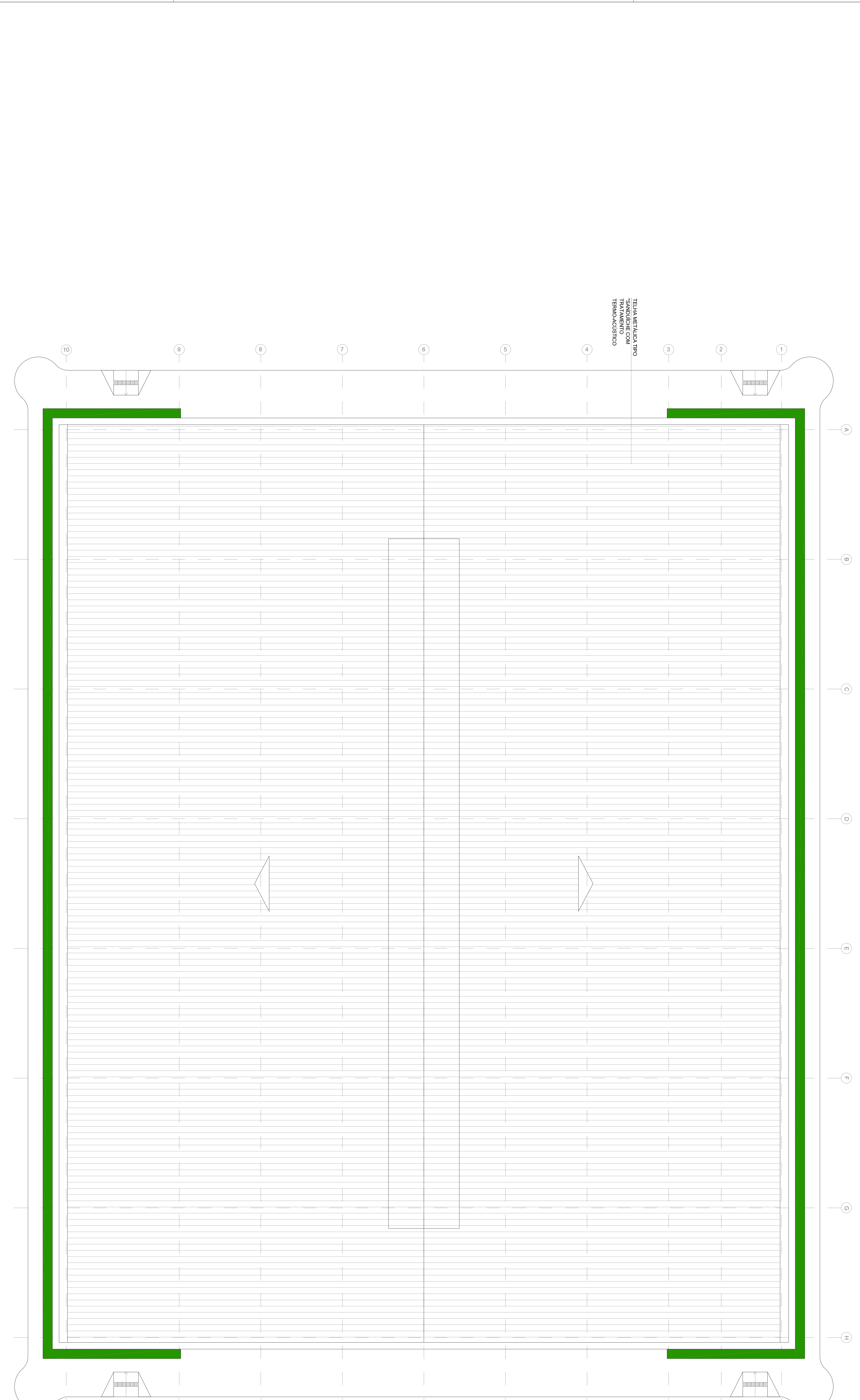
GINÁSIO - PLANTA DE COBERTURA ESC. 1:75
